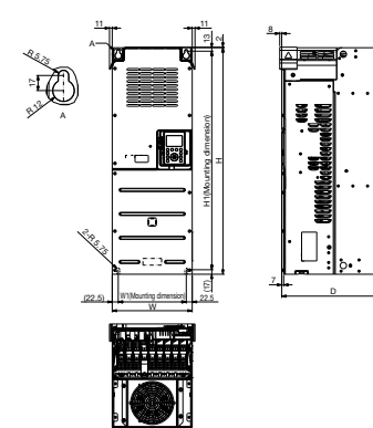
Frame Size A6
