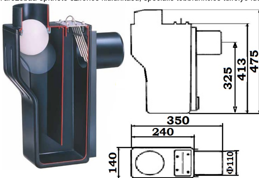
HK MULTISIPHON 100
