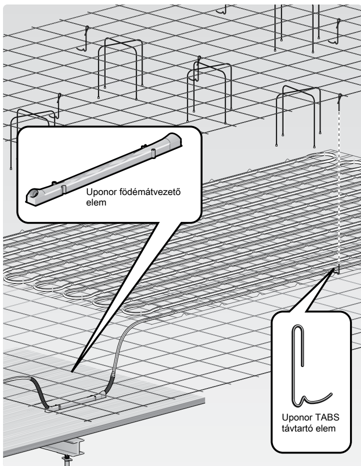
Robbantott ábra egy helyszínen szerelt Uponor TABS rendszerről
