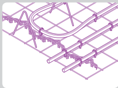
Ipari padlófűtés
