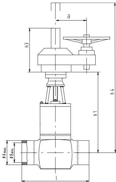
Fig. 5: ≥ DN 600/500
