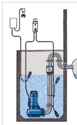
Beépítési javaslat Ama-Porter maximumszint riasztással
