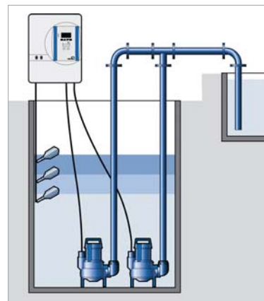
Beépítési javaslat Ama-Porter LevelControl Basic 2-vel
