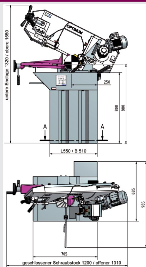
Méretek S 275 G
