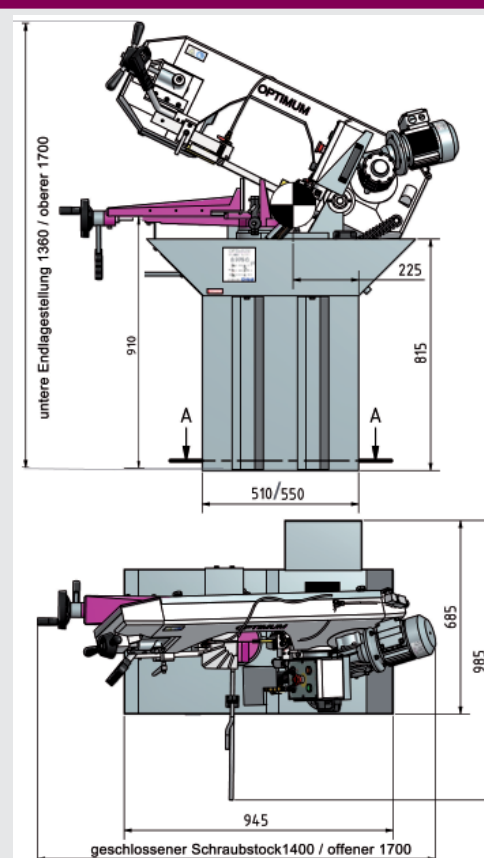
Méretek S 275 G
