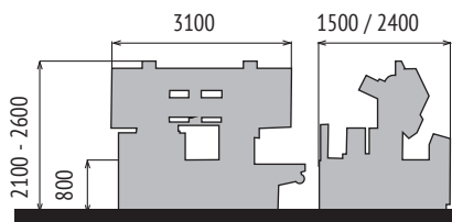
HMBS 510 x 510 HA-FX / CNC-FX méretei
