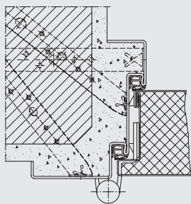
Eckzarge Profil 185 – Ausführung für Mauermontage
