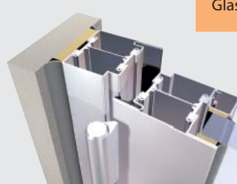
Rohrrahmentürelement
