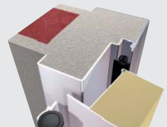
Dünnfalz-Türelement
