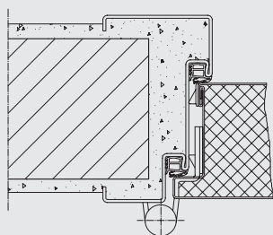
Umfassungszarge Profil 186 – Ausführung für Mauermontage
