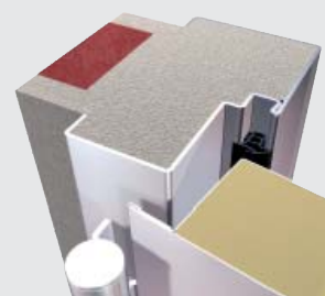
Dünnfalz-Türelement
