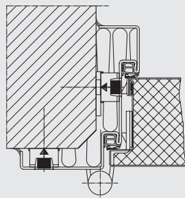
Profil 185 – Ausführung für Dübelmontage
