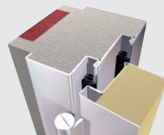
auch bündig einschlagend einbaubar mit Doppelfalzzarge
