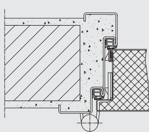
Umfassungszarge Profil 187 – Ausführung für Mauermontage
