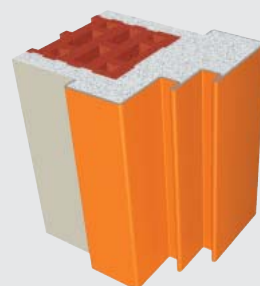
Mauermontage nachträglich
