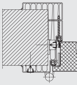
Umfassungszarge Profil 185 + 67 – Ausführung für Dübelmontage
