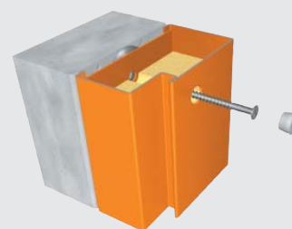
Dübelmontage
