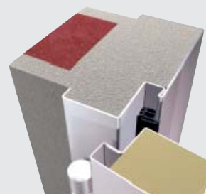
Dickfalz-Türelement in Zarge mit Einfachfalz
