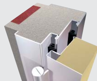
bündig in Doppelfalzzarge einschlagend
