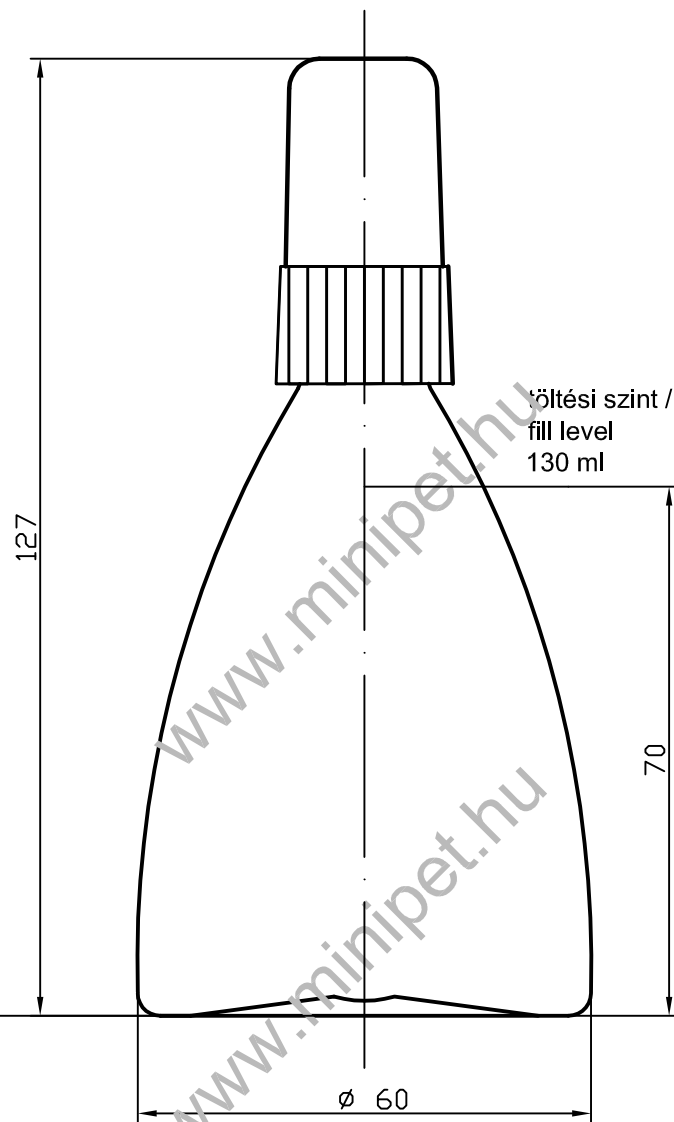
Termék/Product: PET palack/bottle 20/410 szórófejjel/ with 20/410 pump sprayer Típus/Type: Illat130 Menet/Neck: KS20 Súly/Weight: 17 gramm www.minipet.hu
