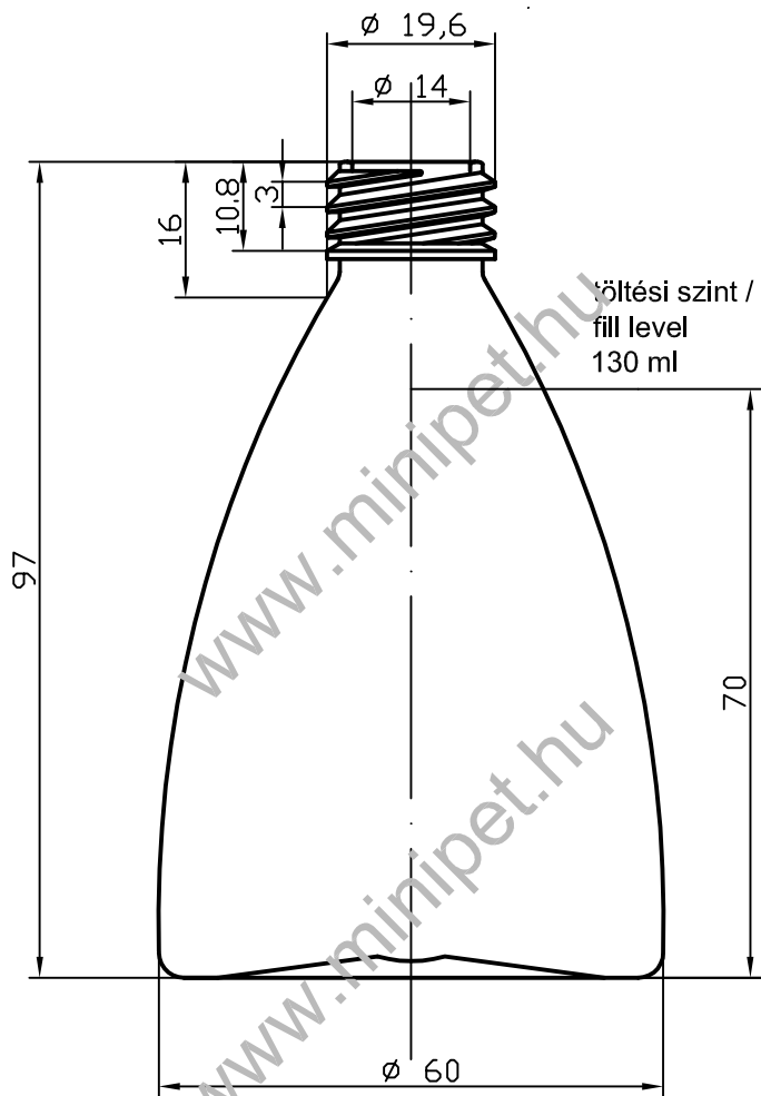
Termék/Product: PET palack/bottle Típus/Type: Illat130 Menet/Neck: KS20 Súly/Weight: 17 gramm www.minipet.hu
