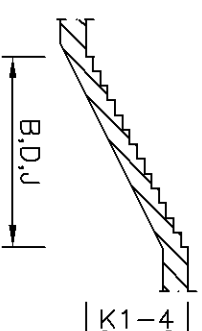
LÉPCSŐKAR METSZET
