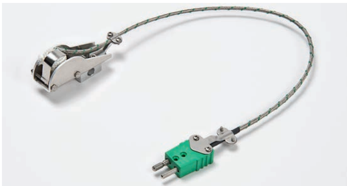
Csúszó hőelem, OS 450
