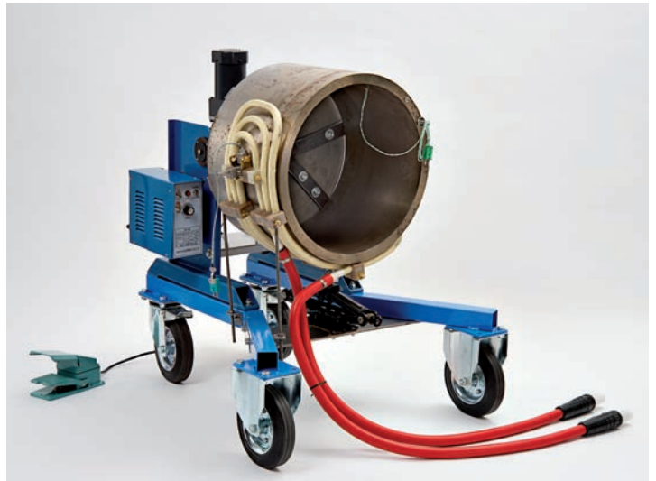
Forgóberendezés rögzített induktorrall
