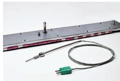
Mágneses előmelegítő bajonettzáras hőelemmel
