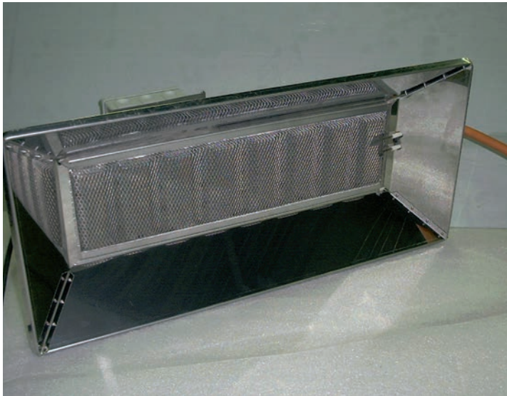
Infravörös gázugárzó reflektorral
