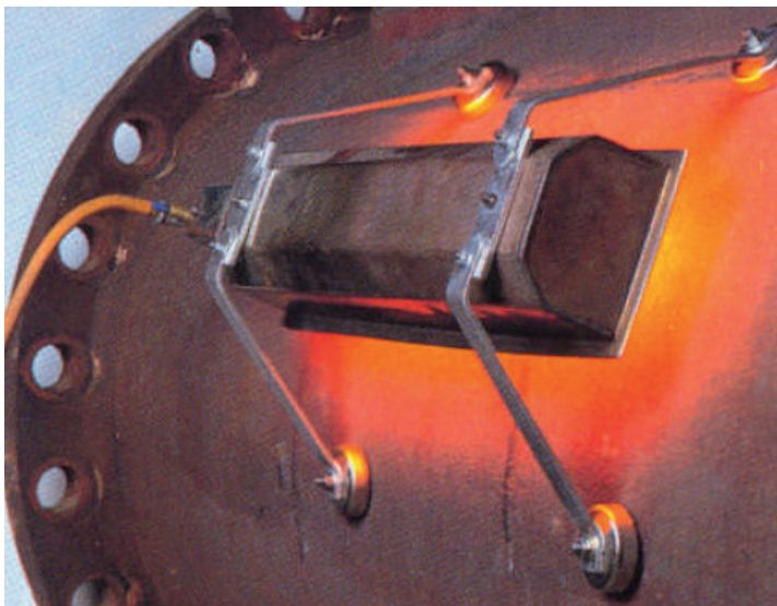
Infravörös gázugárzó a tartályon
