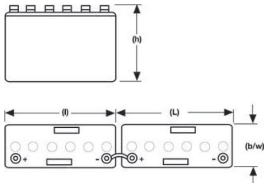
12V 1 OPzS 50 LA — 12V 3 OPzS 150 LA
