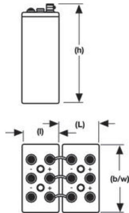
12V 1 OPzS 50 LA — 12V 3 OPzS 150 LA
