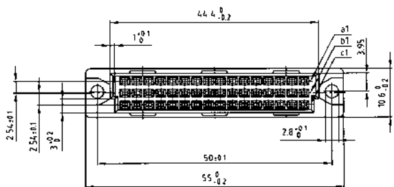
Wire Wrap
