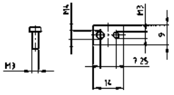
Mounting set for DIN 41617
