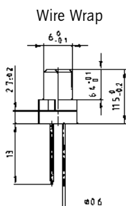
Wire Wrap
