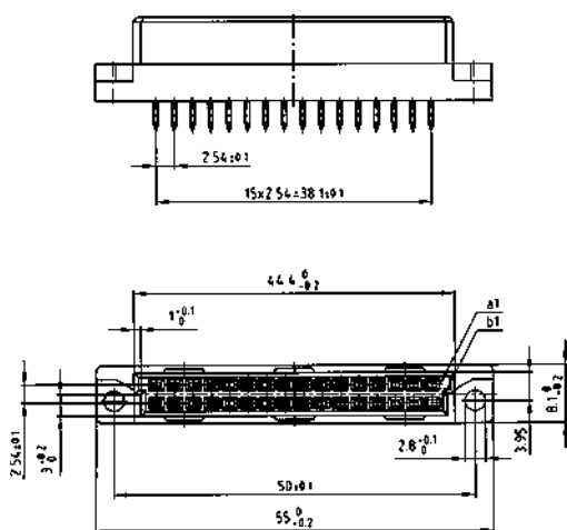
Wire Wrap
