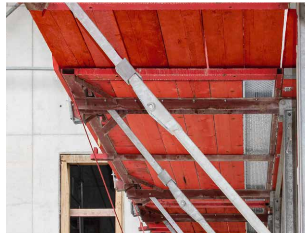
Az állvány kitámasztó rudazata önreteszelő biztosítókkal rendelkezik.
