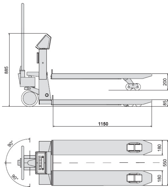
Méretetek mm-ben
