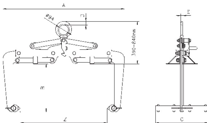
TBA modell: 0,2-1 t bordázott befogópofákkal
