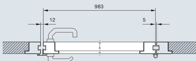
Vízszintes metszet ET 500 billenőkapu személybejáró-ajtóval
