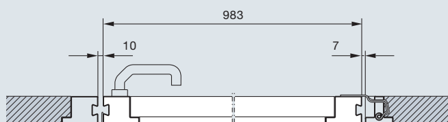
Vízszintes metszet ST 500 tolókapu személybejáró-ajtóval
