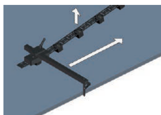
UST-0466-53-00-00-0 Terelőelem állító eszköz a sín éllel való párhuzamos beállításához
