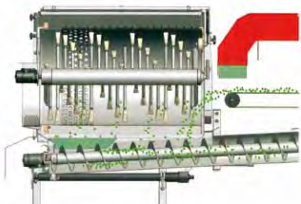
A bogyózó kapacitása nagy szüretelési sebességet tesz lehetővé nagy terhelés mellett is.
