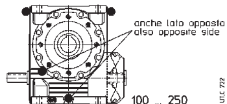
Forma costruttiva - Mounting position B6 1)
