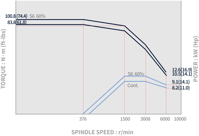
Main spindle_ Lynx 2100A / LA / MA / LMA / LMSA
