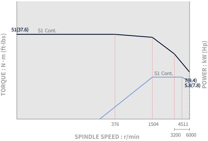
Sub spindle_ Lynx 2100LMSA / LMSB
