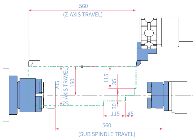
OD HOLDER
