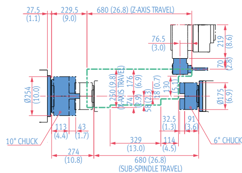
ANGULAR MILLING HOLDER (SUB)
